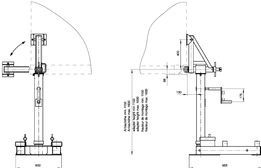
Typ(e) 3108 Weitere Darstellungen finden Sie auf www.haacon.com unter der Produktkategorie „Abstellvorrichtungen“. You find further drawings on www.haacon.com under the product category 'Container support devices'. Vous trouvez d'autres dessins sur www.haacon.com sous la catégorie de produit « Support de conteneur ».
